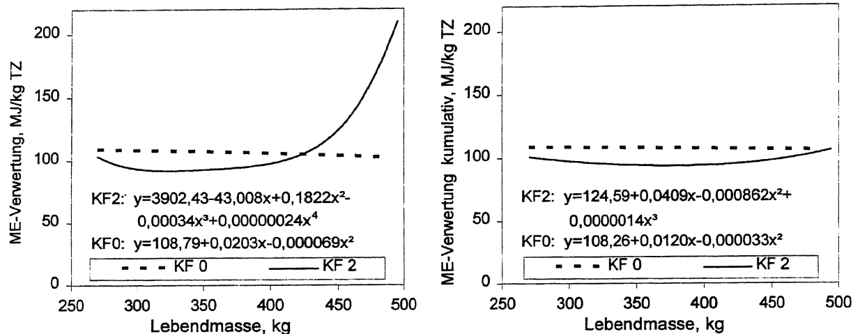
Abbildung 5: Verlauf der Energieverwertung und der kumulativen Energieverwertung Figure 5: Energy efficiency and cumulative energy efficiency depending on live weight
