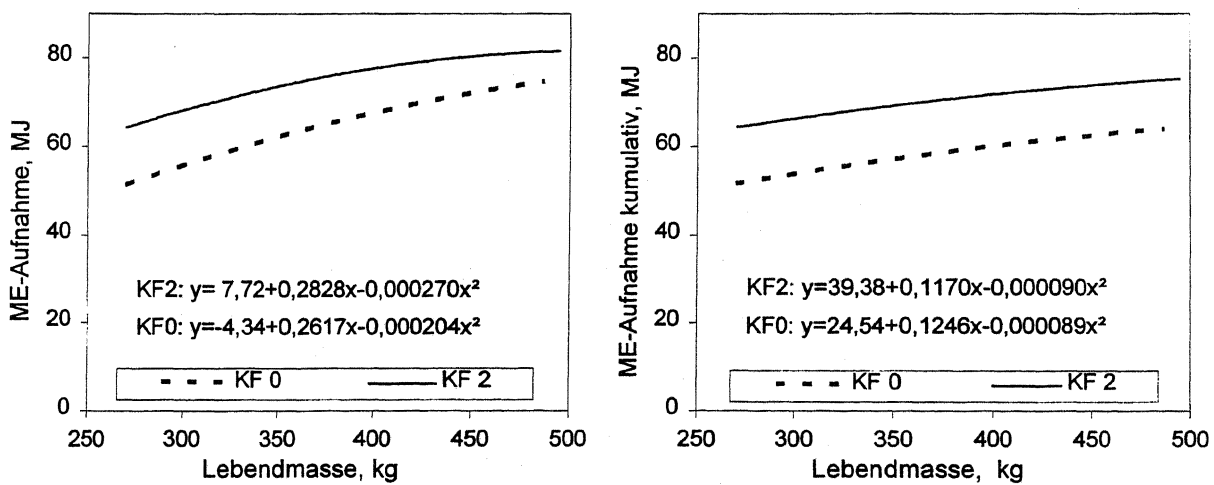
Abbildung 4: Verlauf der Energieaufnahme und der kumulativen Energieaufnahme Figure 4: Energy intake and cumulative energy intake depending on live weight
