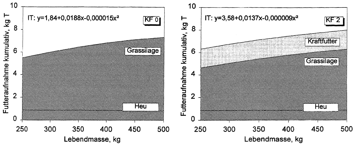
Abbildung 2: Verlauf der kumulativen Futtermittelaufnahme Figure 2: Cumulative feed intake depending on live weight
