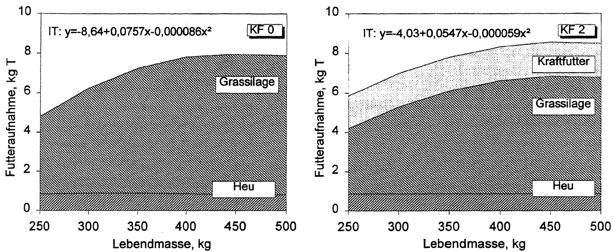
Abbildung 3: Verlauf der Futtermittelaufnahme Figure 3: Feed intake depending on live weight
