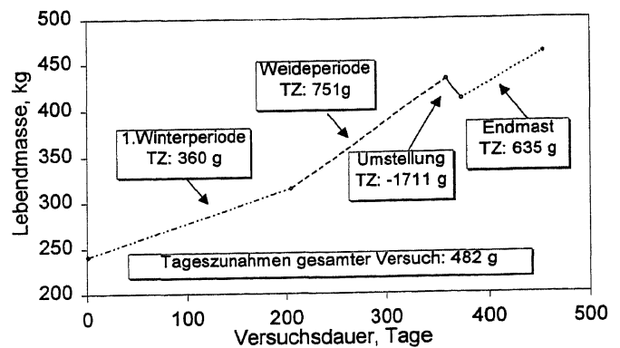
Abbildung 6: Entwicklung der Lebendmasse im Extensivmastversuch Figure 6: Live weight development in the extensive feeding trial
